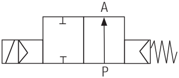
Funktion NO (Ventil in Ruhestellung geöffnet)
