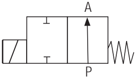
Funktion NO (Ventil in Ruhestellung geöffnet)
